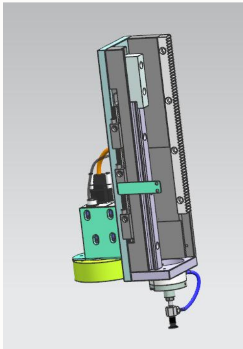
x轴模组装配体
